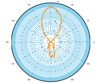
5.5 Ghz H-Plane and E of H-plane
