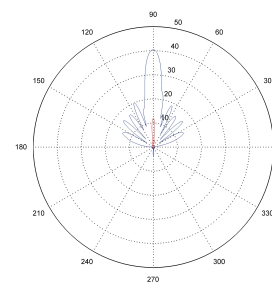
5.5 Ghz H-Plane and E of H-plane
