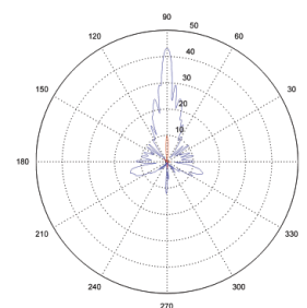
5.5 Ghz H-Plane and E of H-plane
